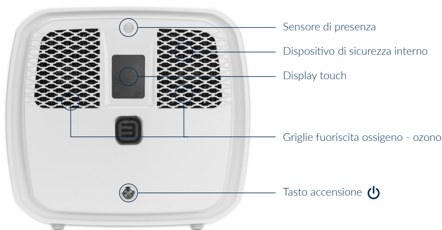
VISTA FRONTALE
