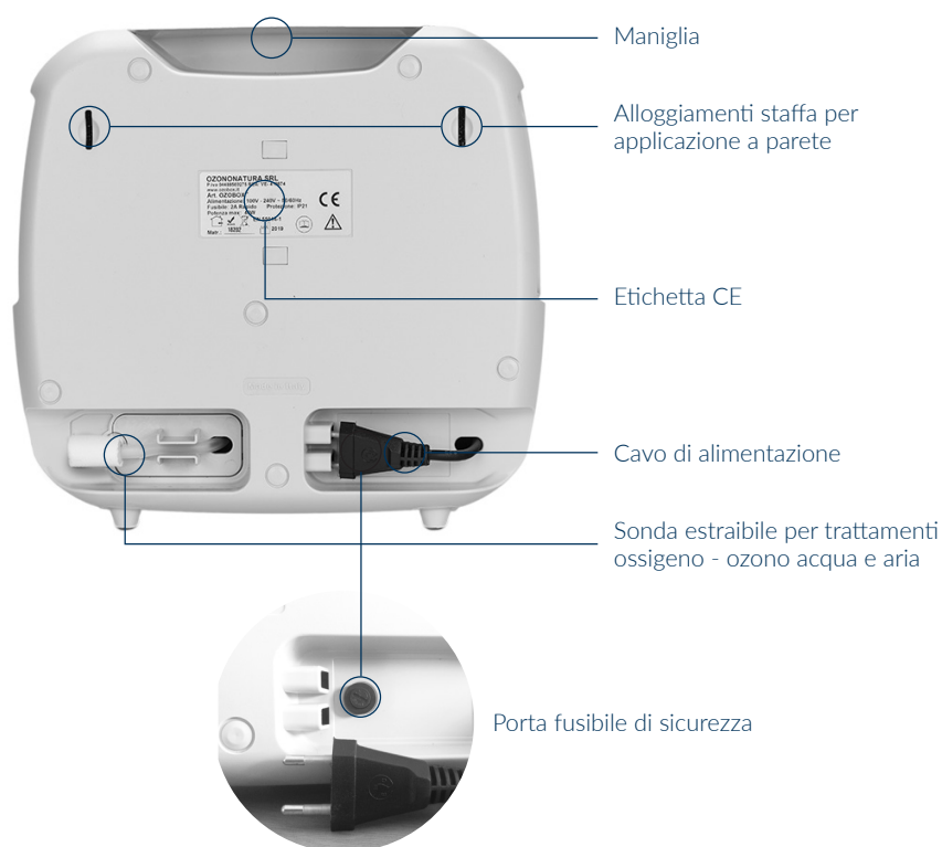
VISTA POSTERIORE
